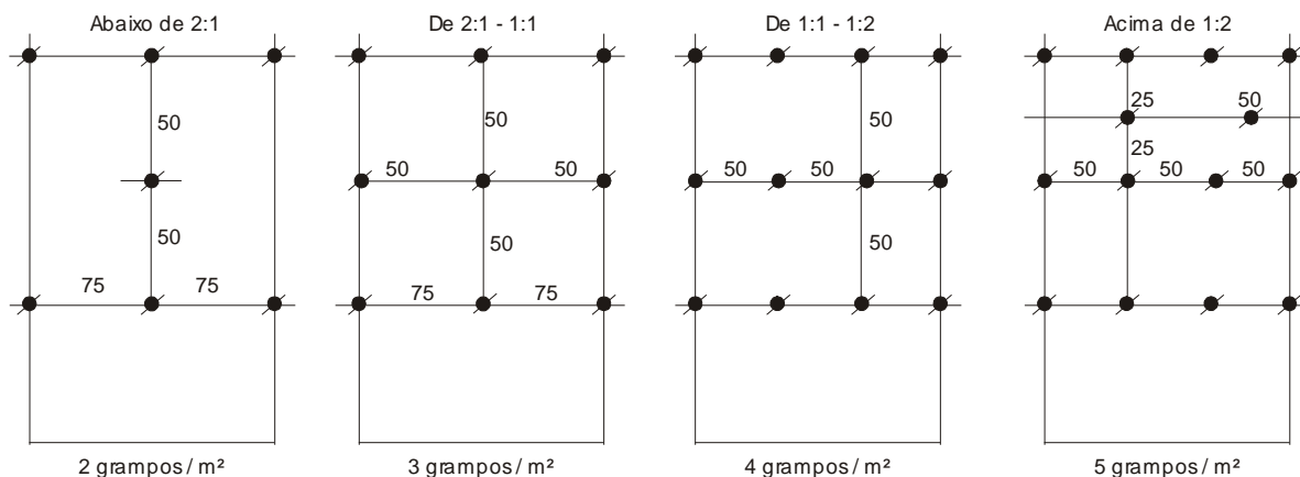
FIGURA 3.2.9-6 - Fixação de biomantas de acordo com a inclinação dos taludes
