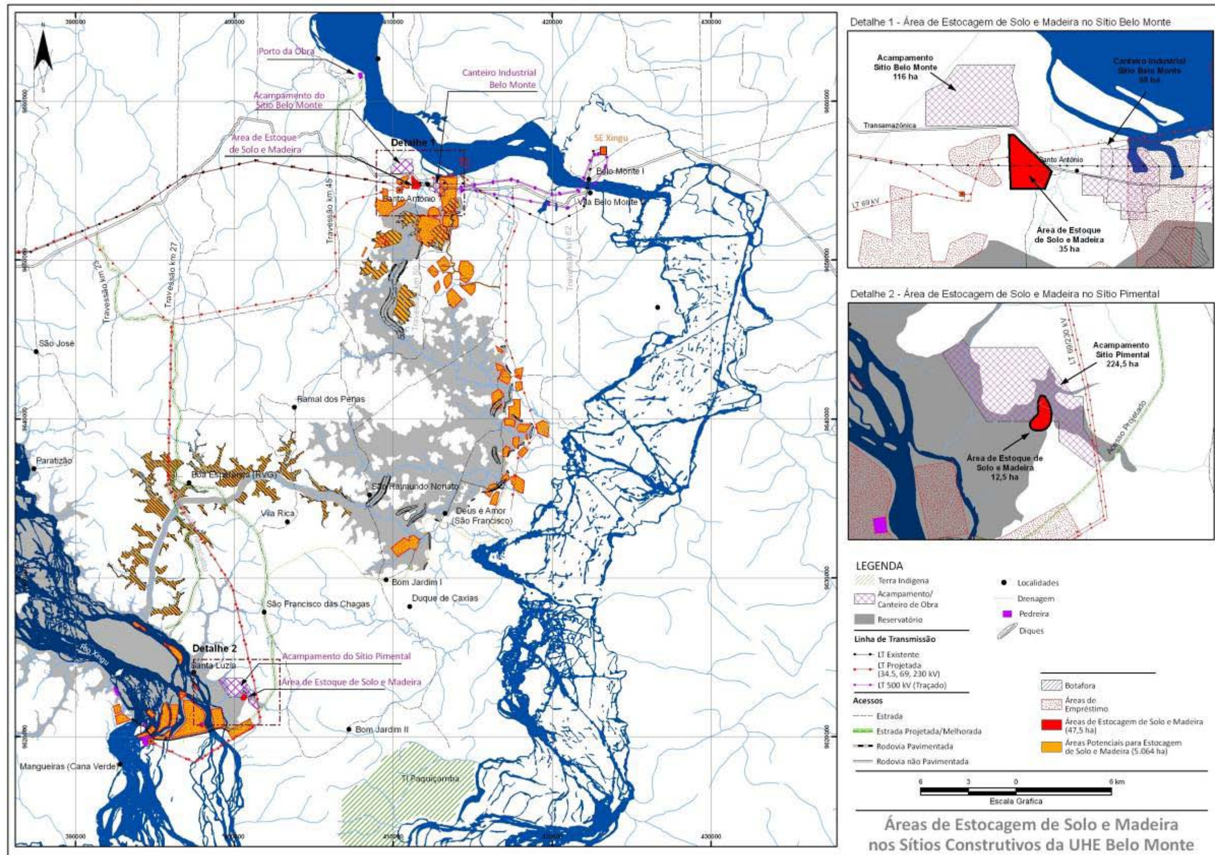
FIGURA 3.2.9-1 - Áreas de estocagem de solo e madeira nos sítios construtivos da UHE Belo Monte
