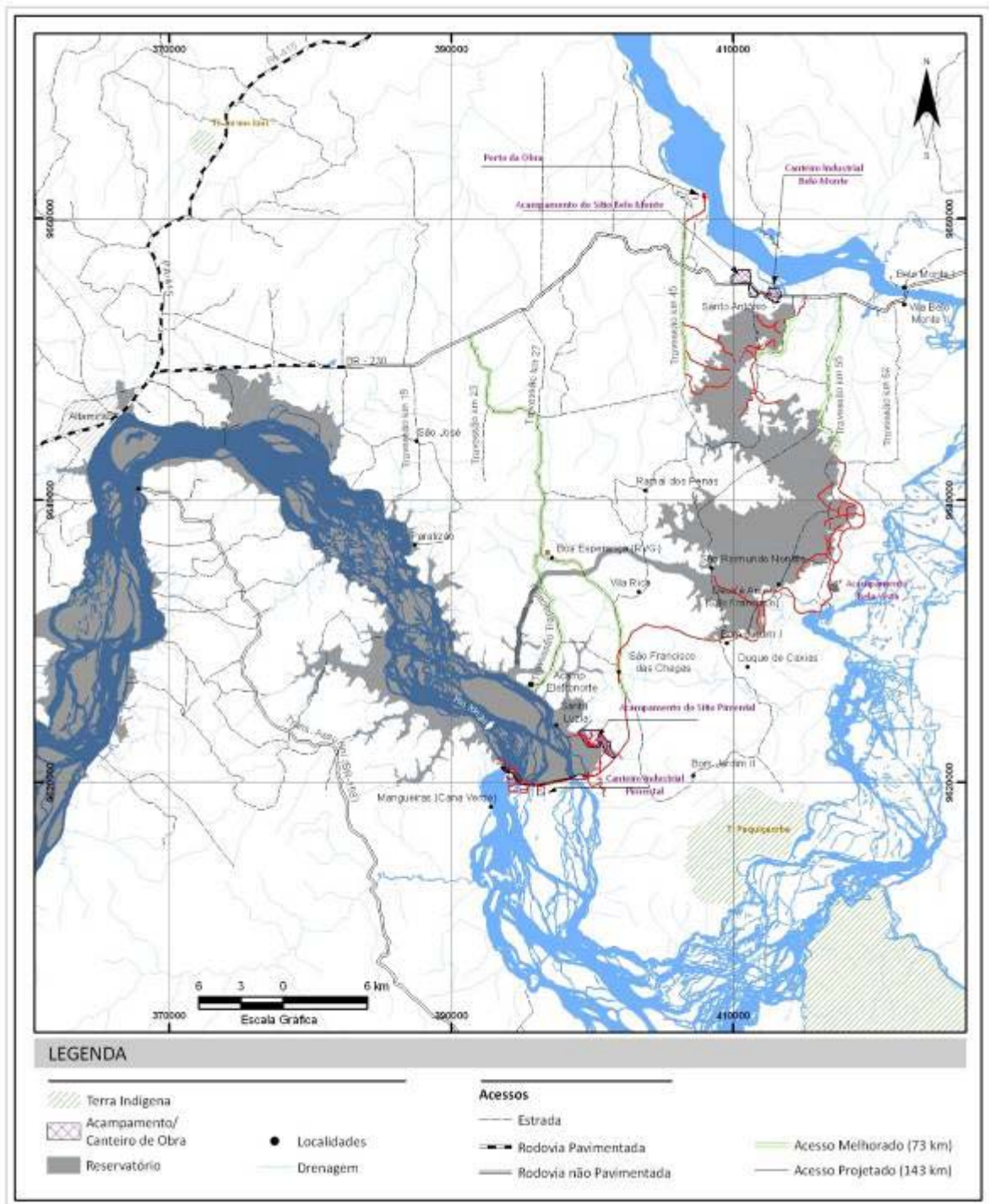
FIGURA 3.2.9-5 - Rede viária para implantação da UHE Belo Monte
