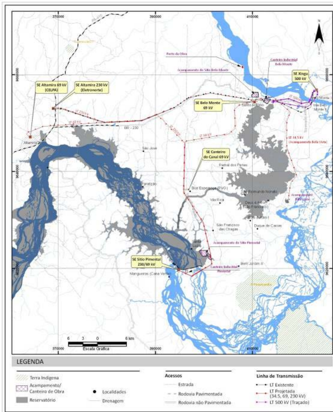
FIGURA 3.2.9-3 – Localização das Linhas de Transmissão e Subestações.
