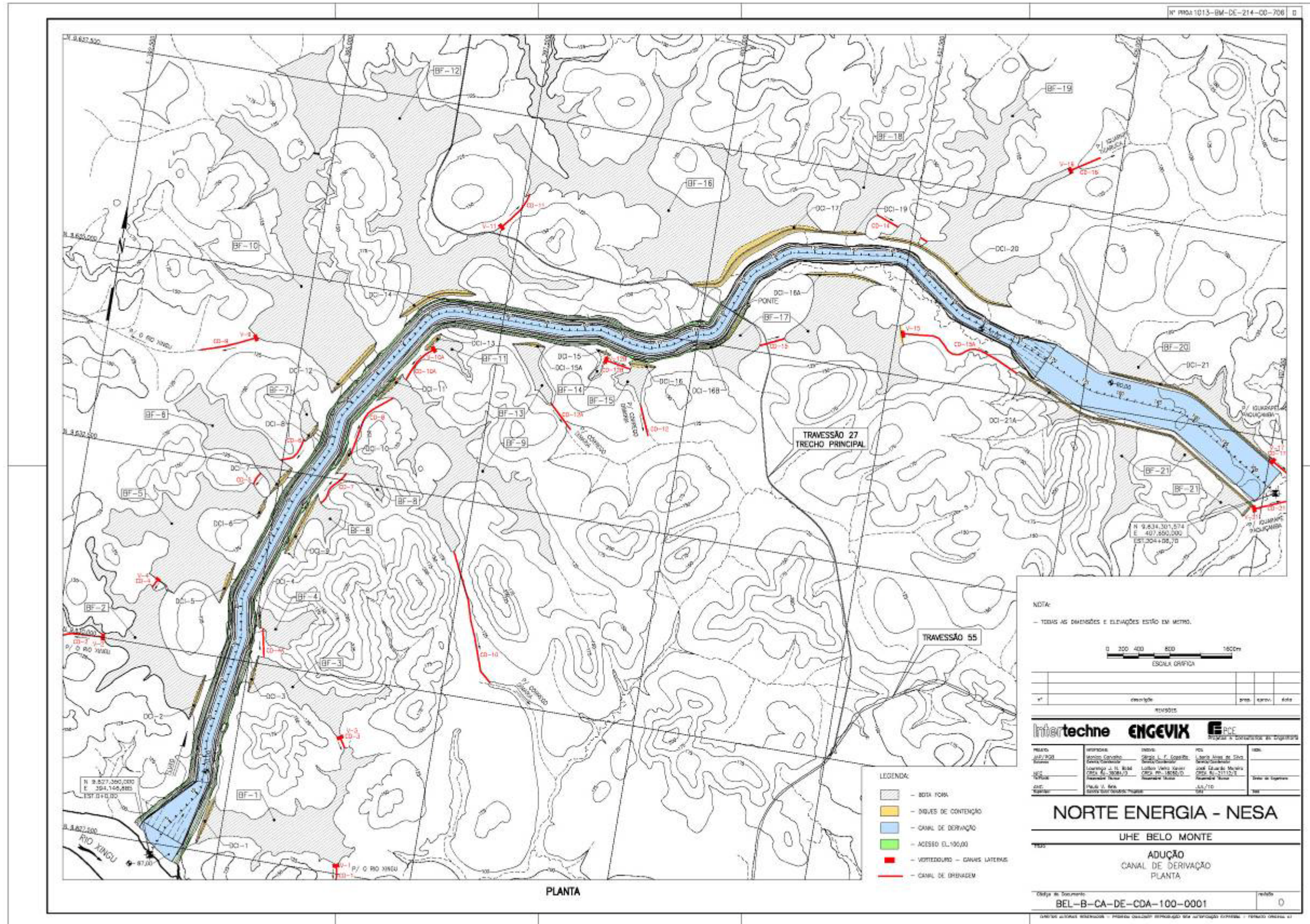
FIGURA 3.2.9-8 – Desenho BEL-B-CA-DE-CDA-100-0001 – Adução – Canal de Derivação
