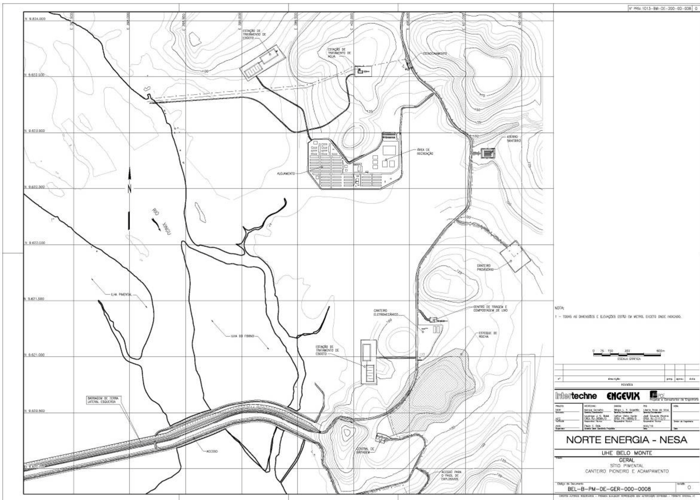
FIGURA 3.1.1-1 - Canteiro Pioneiro e Acampamento do Sítio Pimental
